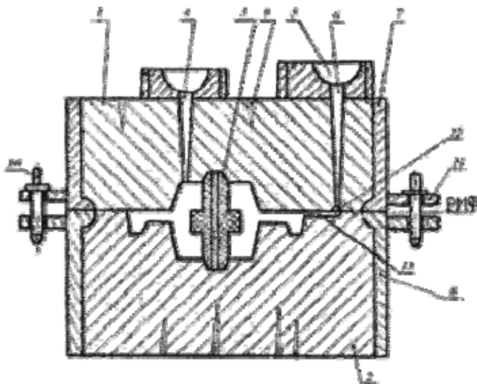
Рис. 2. Литейная форма
